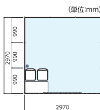
パラペット/スリットタイプ (色はシルバーです)
